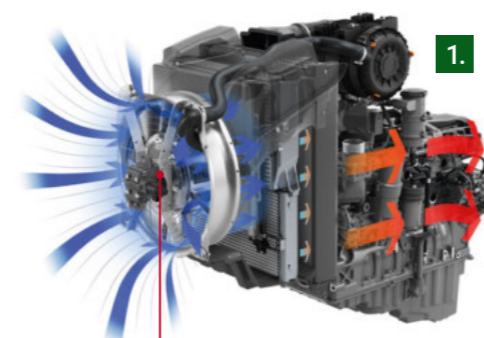
Hydraulic fan drive
